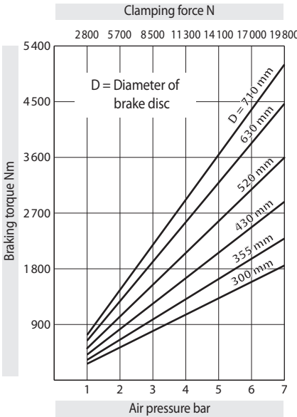
Brake Caliper DV 035 PFM - 660
