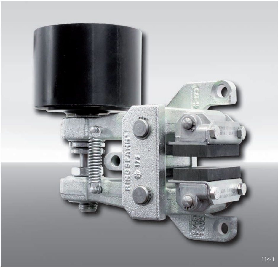
Brake Caliper DH 030 PFM - 635
