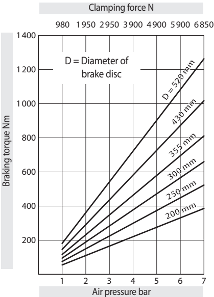
Brake Caliper DH 025 PFM - 635
