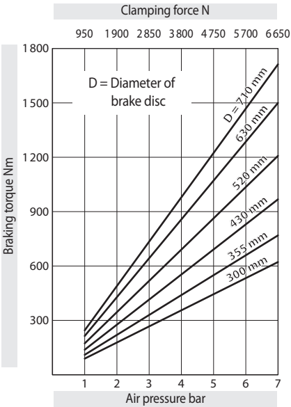
Brake Caliper DH 035 PFM - 635
