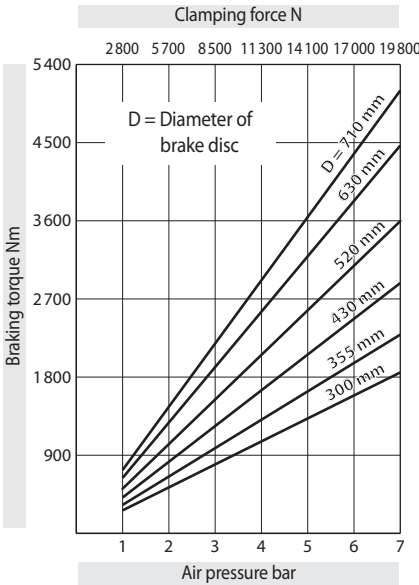
Brake Caliper DH 035 PFM - 660
