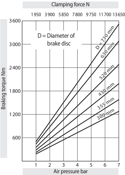
Brake Caliper DH 035 PFM - 655
