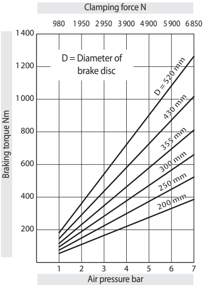
Brake Caliper DV 030 PFM - 635
