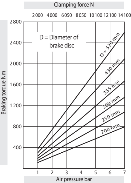
Brake Caliper DH 030 PFM - 655
