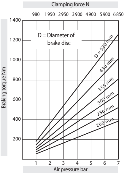
Brake Caliper DH 030 PFM - 635
