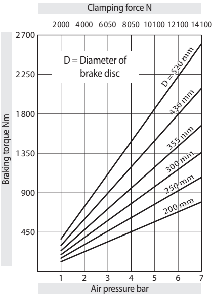
Brake Caliper DH 025 PFM - 655
