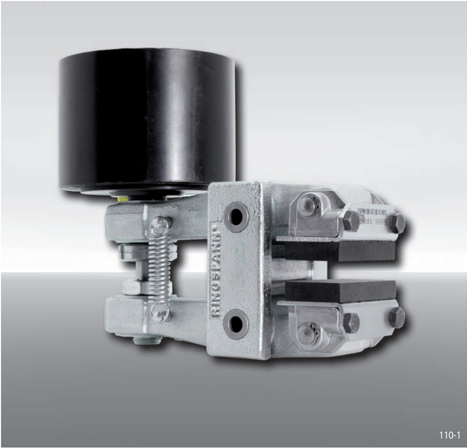
Brake Caliper DH 025 PFM - 635
