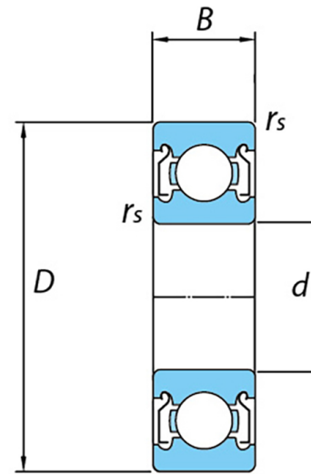
Shielded type (ZZ)
